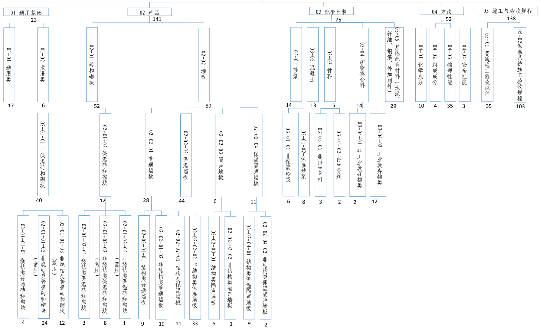
江苏省环境友好墙体材料标准体系结构图
